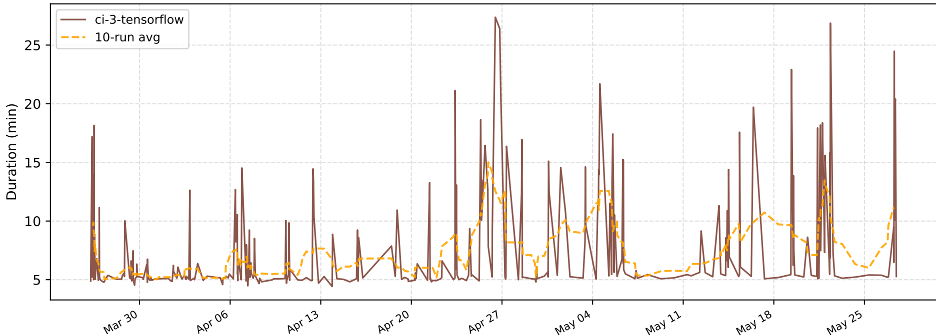
ci-3-tensorflow
